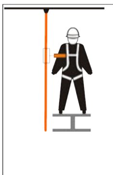
Meelopende valbeveiliging met bewegende geleiding
