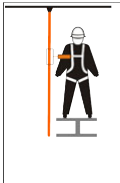
Antiquedas do tipo guiado, incluindo um cabo flexível de ancoragem
