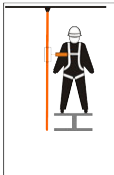
Styrt glidlås med flexibel förankringslina
