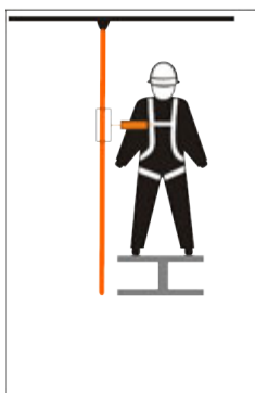
Medløpende fallsikringsenhet med bevegelig føring
